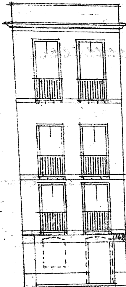
PROSPETTO
