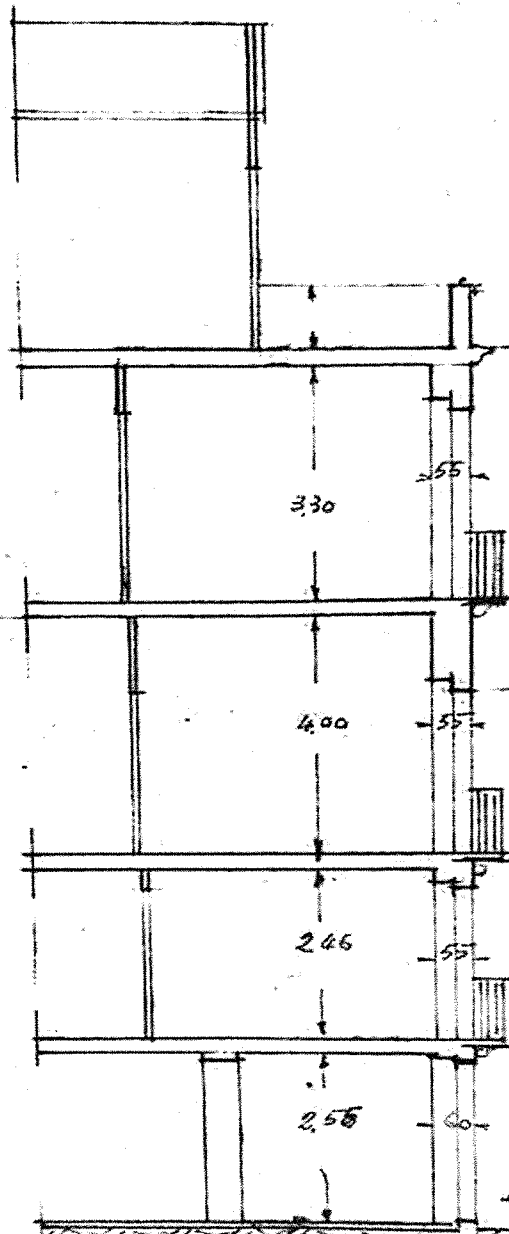
SEZIONE
